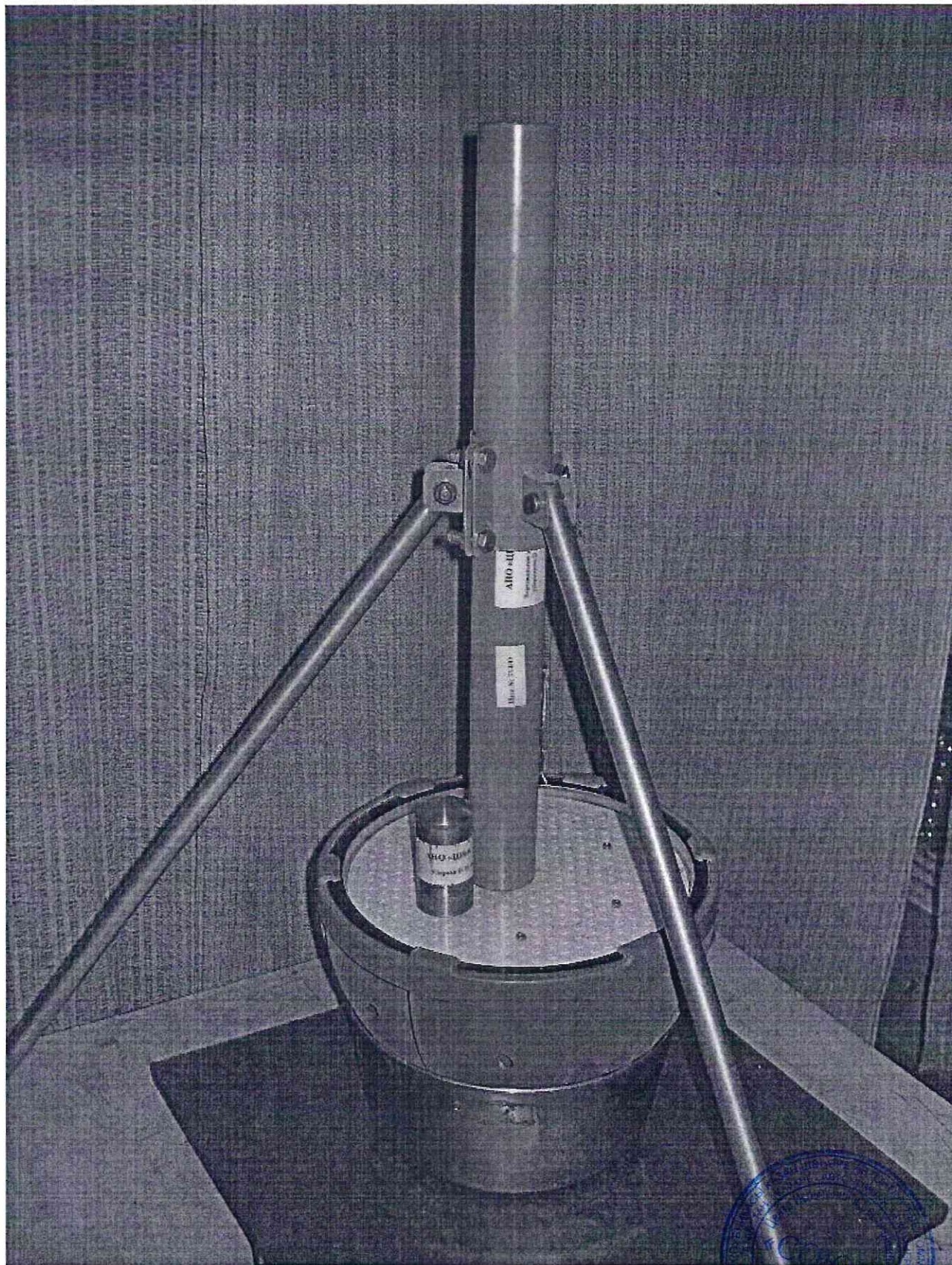
Рис. 3. Вид на вертикальное ударное устройство ВУУ-2 с ударником D-35 мм перед испытаниями на ИЖ07
