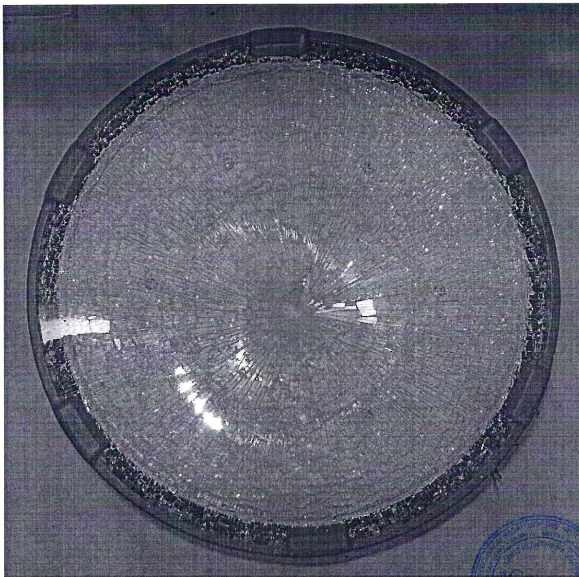
Рис. 7. Вид на светопропускающую часть (рассеиватель) светильника после испытаний на ИК09
